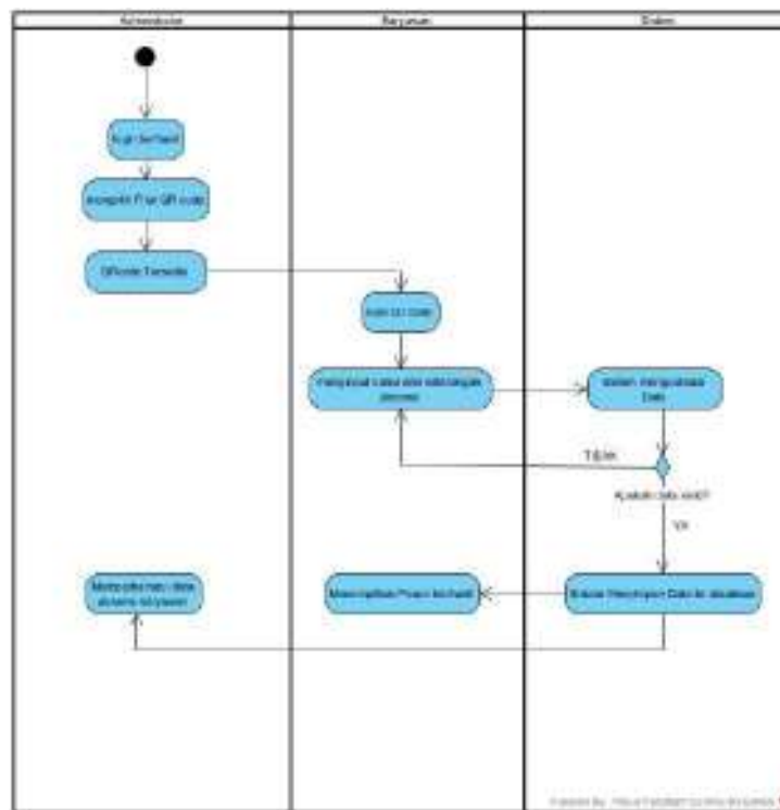
Gambar 5.20 Activity Diagram Absensi Karyawan dengan QR code
