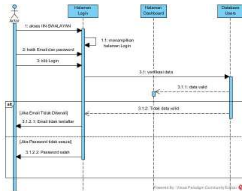
Gambar 5.5 Sequence Diagram Autentifikasi Admin
