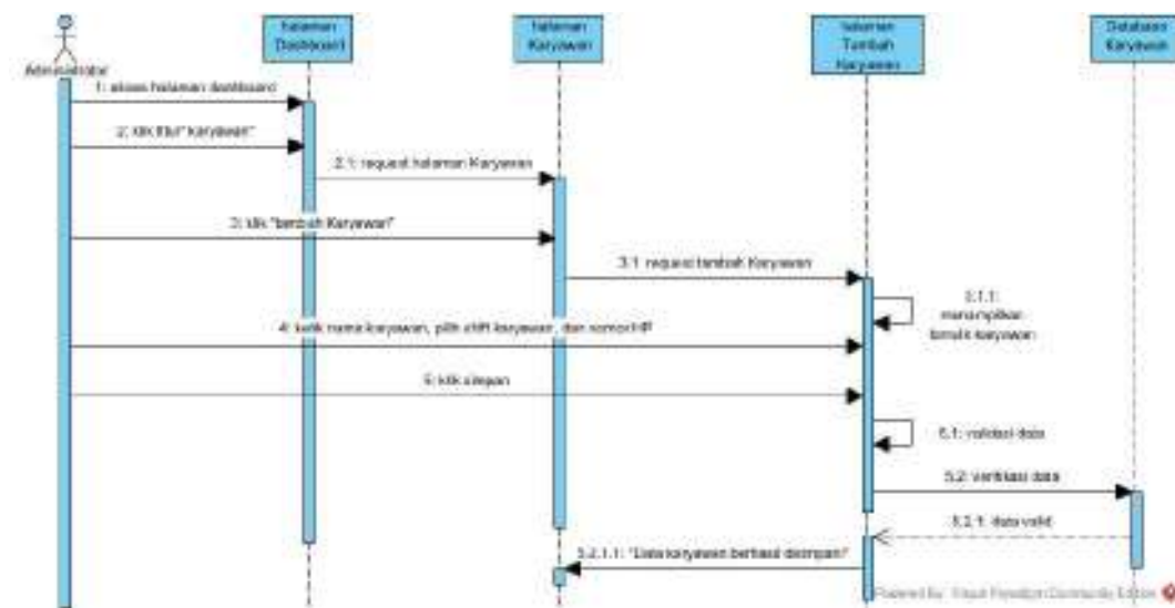
Gambar 5.6 Sequence Diagram Manajemen Karyawan (tambah karyawan)
