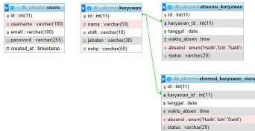
Gambar 5.22 Rancangan Basis Data Sistem Absensi Karyawan
