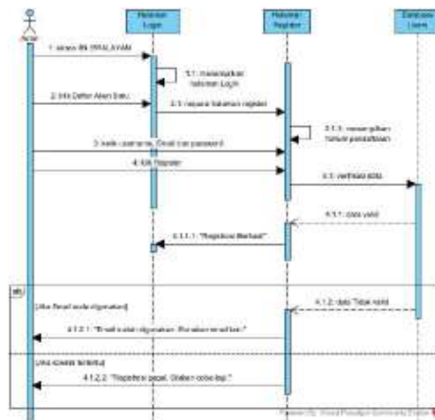
Gambar 5.4 Sequence Diagram Autentifikasi Admin A-1(Registrasi Admin)
